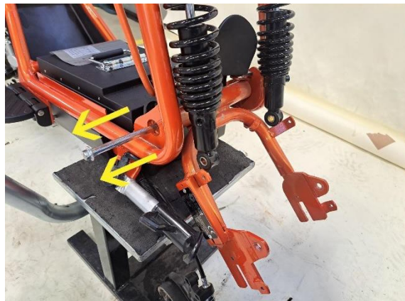
Vedä takahaarukan akselipultti pois.
