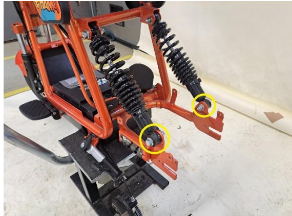
Irrota takajousien alapäiden kiinnityspultit (kiintoavain 14 mm).
